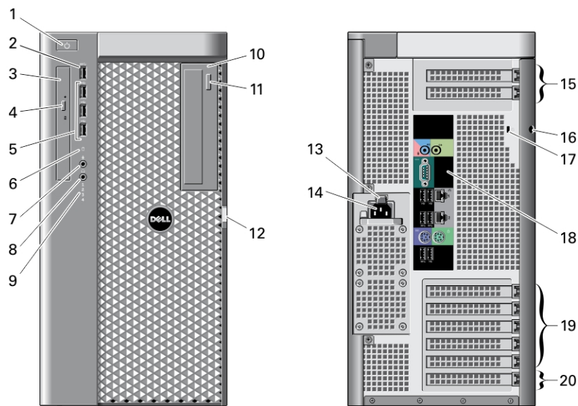
Slika 3. Pogled s prednje i stražnje strane T7610 računala
