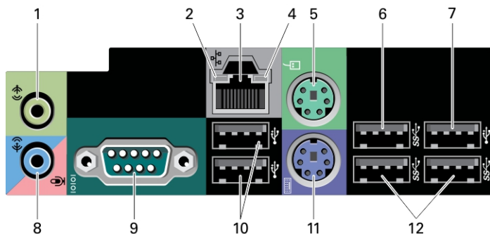
Slika 2. Pogled na stražnju ploču T3610/T5610 računala
