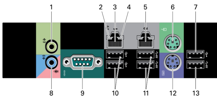
Slika 4. Pregled stražnje ploče
