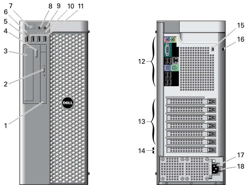
Slika 1. Pogled s prednje i stražnje strane T3610/T5610 računala
